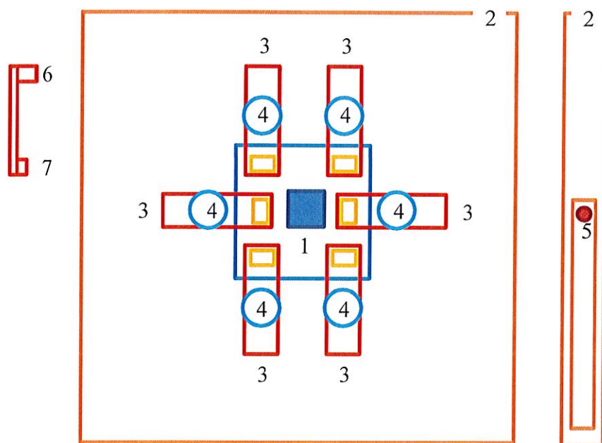
Rys. 1. Schemat układu zasilania i układu mocowania LED.
